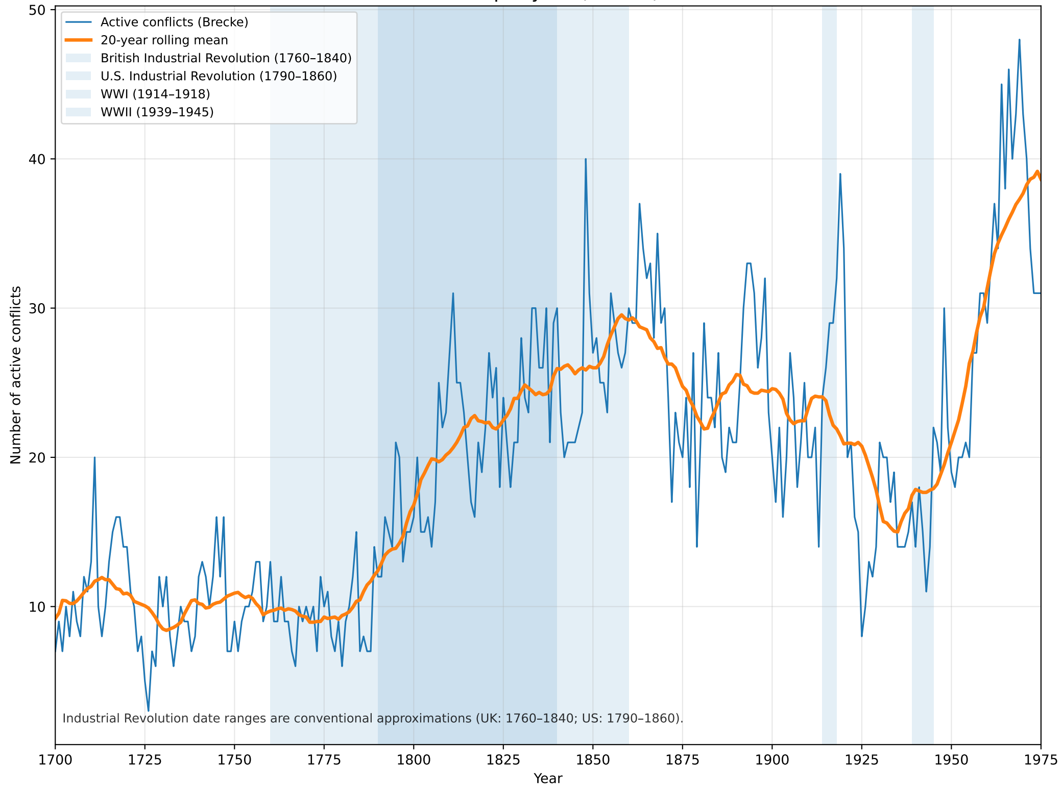
A: Active conflicts per year (Brecke), 1700-1975
